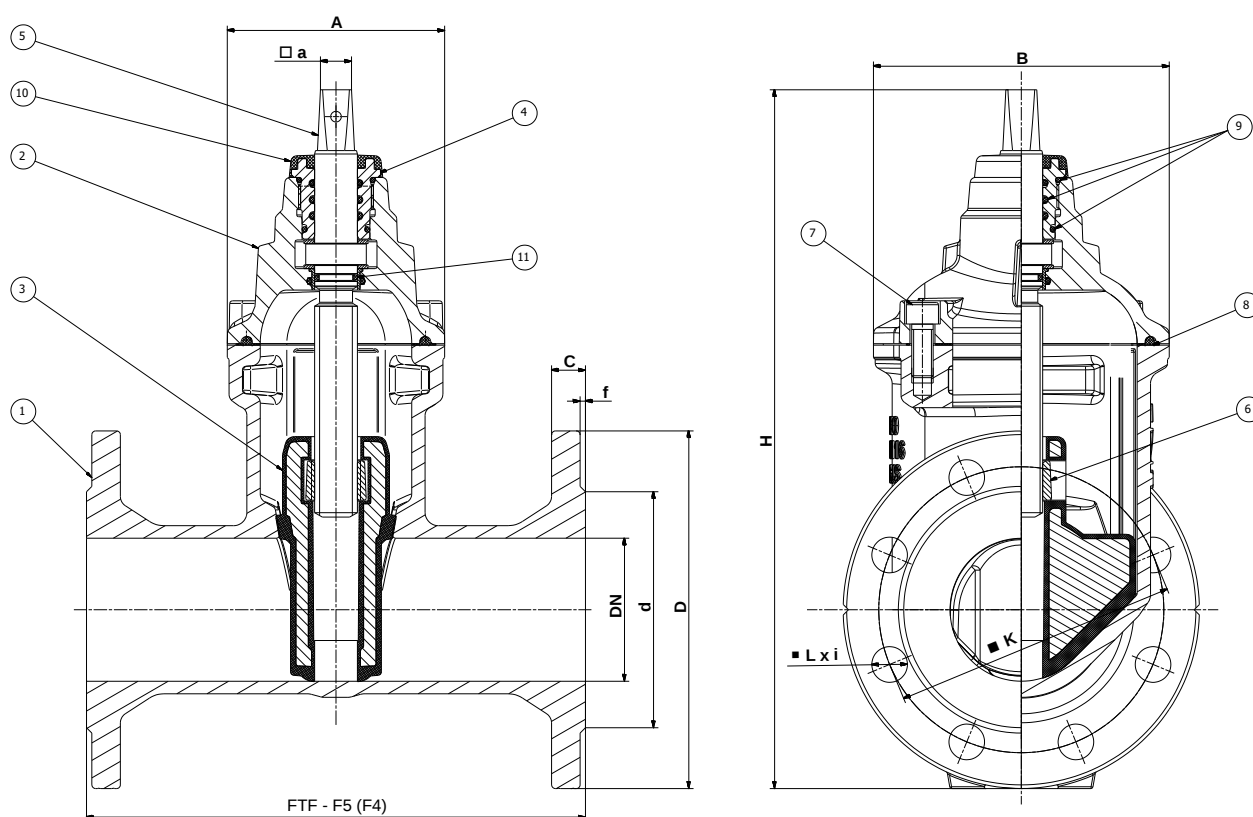
Rys. 1 – Budowa zasuwy kołnierzej z miękkim uszczelnieniem
