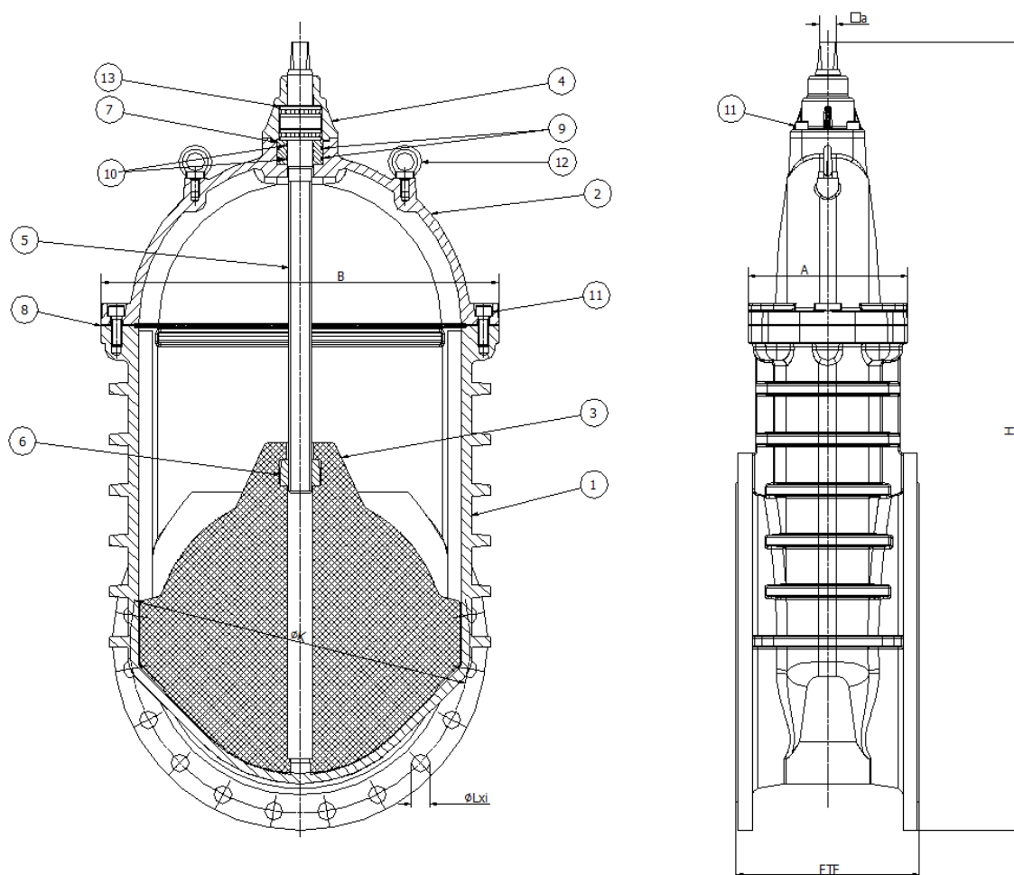
Rys. 1 – Budowa zasuw zaporowej
